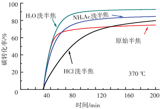
图 5 化学分馏各步半焦 370 °C 下碳转化率曲线
