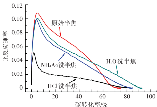
图 6 化学分馏各步半焦比反应速率曲线
