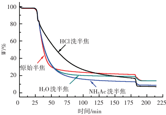
图 3 化学分馏各步半焦反应活性的 TG 曲线
