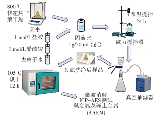
图 2 生物质热解半焦化学分析分馏系统
