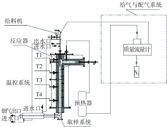
图 1 携带流反应器系统
