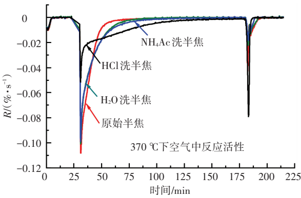
图 4 化学分馏各步半焦反应活性的 DTG 曲线
